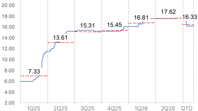
Bismuth(USD/lb)
