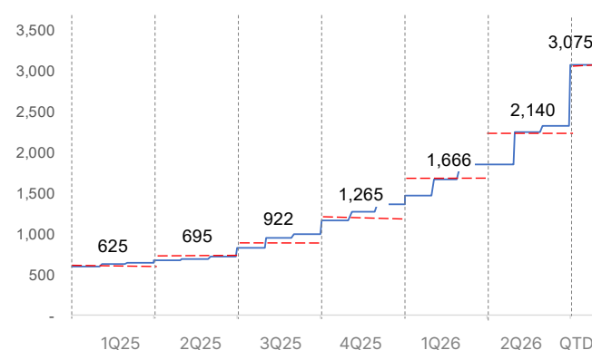
Gallium(USD/kg)
