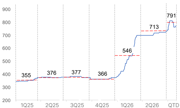
Indium(USD/kg)
