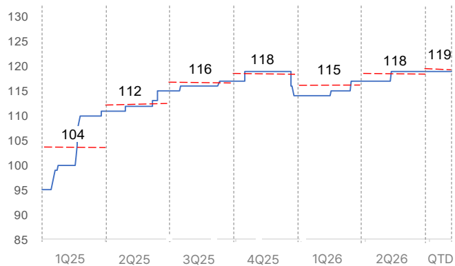
Tellurium(USD/kg)
