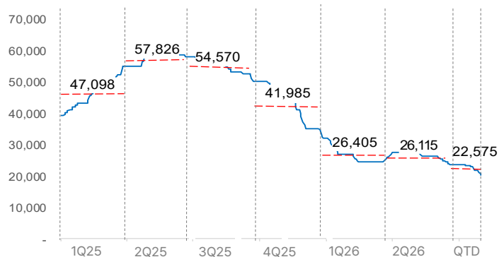
Antimony(USD/MT)
