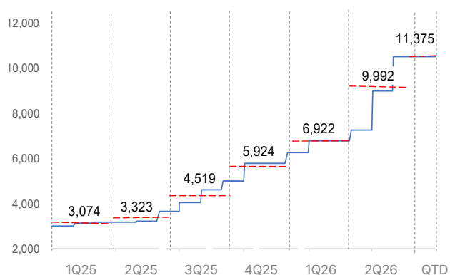
Germanium(USD/kg)
